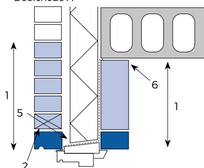
Doorsnede A
