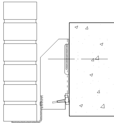
Stelbout niet correct, scheef tegen vloerrand. Recht tikken zoals in vorig plaatje.
