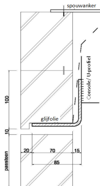
Afb. B Geveldrager t.p.v. horizontale dilatatie
