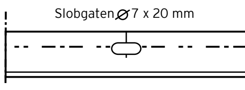
Gaten in bodemplaat
