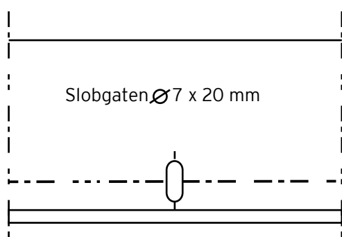
Gaten in hoeklijn GD of LA
