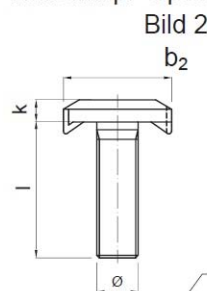
Hakenkopf- Spezialschraube
