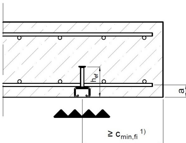
Bild 1: Einseitige Brandbeanspruchung
