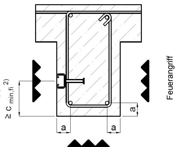
Bild 2: Mehrseitige Brandbeanspruchung
