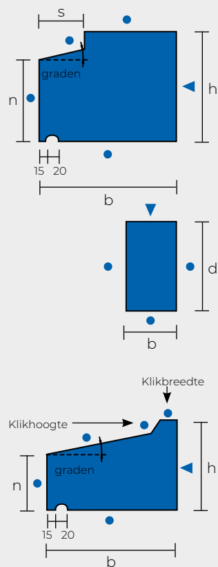
Kozijnkadergevelband (KKG)
