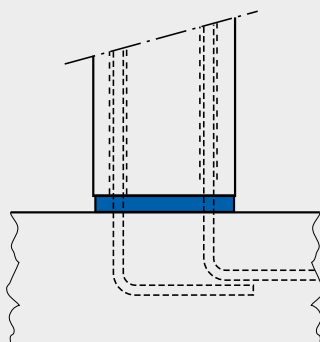
OS-mortel
