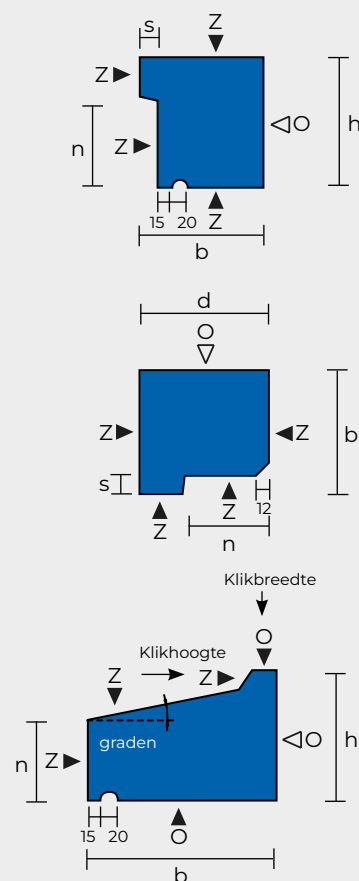
Kozijnkadergevelband (KKG)
