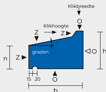
Kozijnkadergevelband (KKG)
